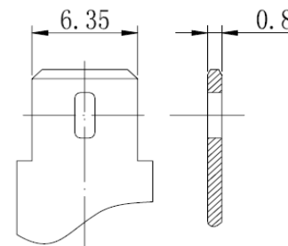
Клеммы
